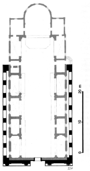
Leon Battista Alberti. Tempio Malatestiano. Pianta. Rimini.
